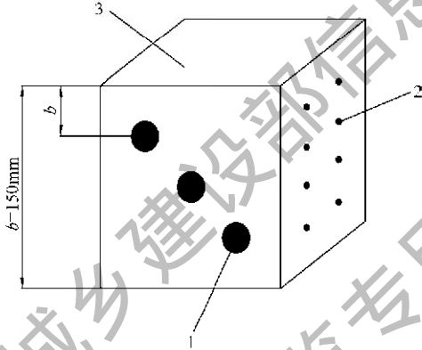
图 C.0.3 声时测量测点布置示意
