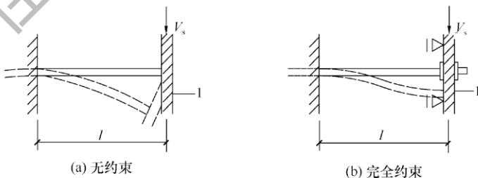
图 6.1.14-2 约束状况示意
