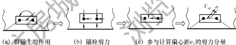
图 5.3.8-3 扭矩与剪力共同作用，
