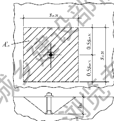
图 6.1.4 理想锥体破坏投影面面积示意
