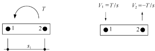
(b) 分配到各锚栓上的剪力
