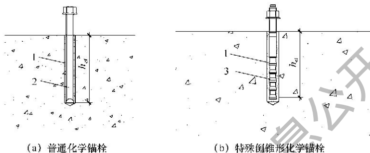
图 A.1.4 化学锚栓示意
