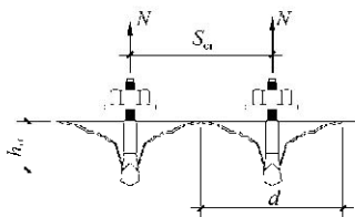
图 A. 2. 2 混凝土锥体受拉破坏示意
