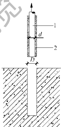
图 A.2.10 普通化学锚栓胶混 界面破坏示意
