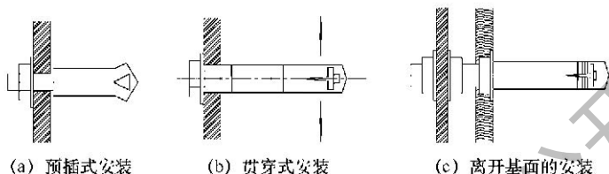
图 9.2.1 锚栓安装方式示意
