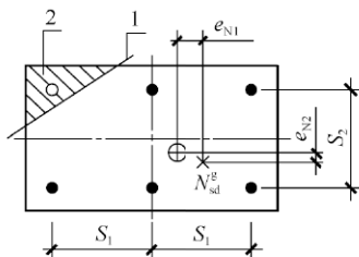
图 5.2.4-3 群锚双向偏心受拉示意
