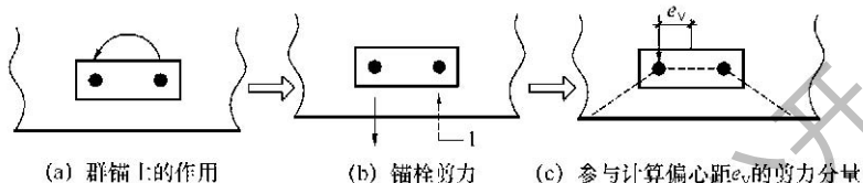
图 5.3.8-1 仅有扭矩作用示意
