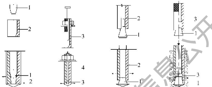
(a) 锥下型(内塞) (b) 杆下型(穿透式) (c) 套下型(外塞) (d) 套下型(穿透式)
