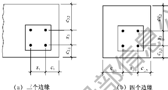
图 6.2.12 有多个边缘影响的群锚示意
