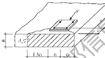
图 6.1.18-3 四栓受剪，位于构件角部示意
