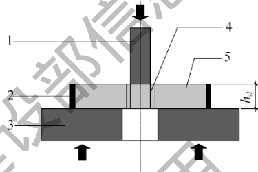
图 B. 1. 17 冲击测试示意
