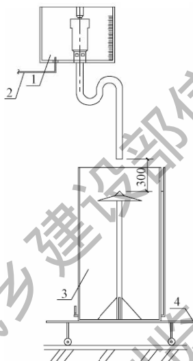
图 B.0.2-1 瞬间流发生器特性测试装置示意图
