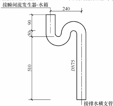
(c) 瞬间流发生器-排水管构造图
